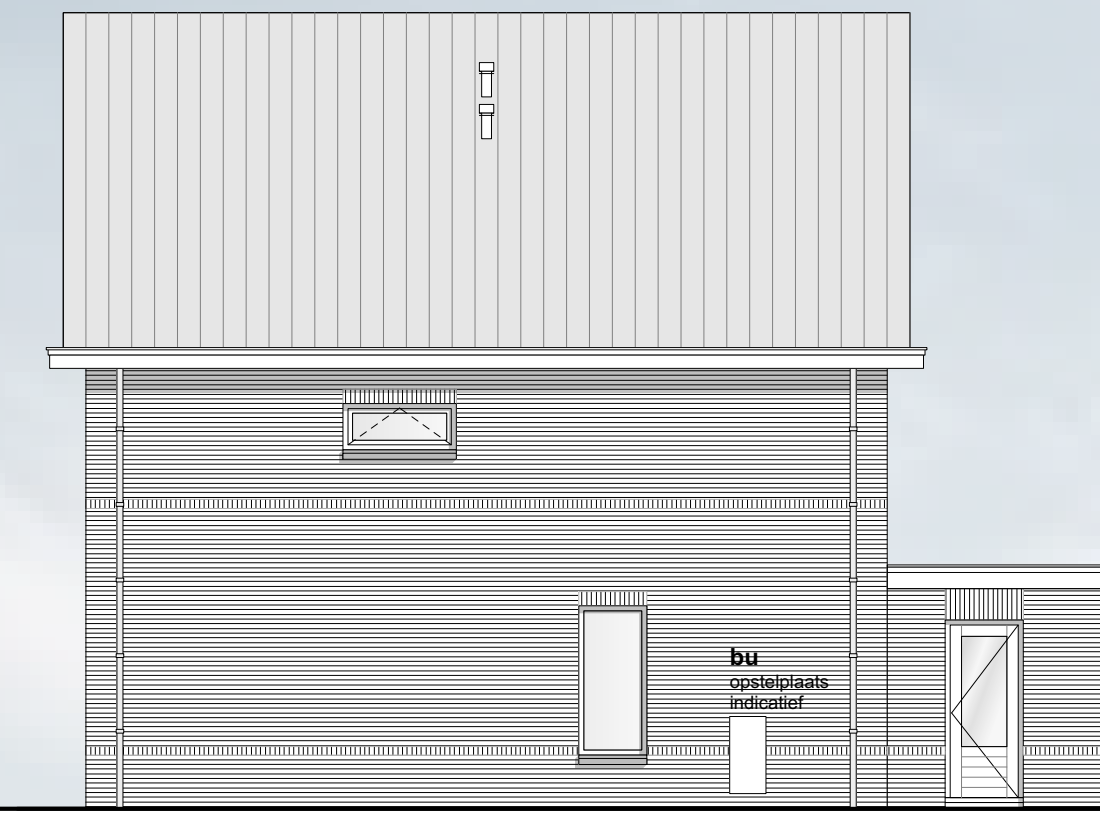
RECHTERZIJGEVEL 1:100
