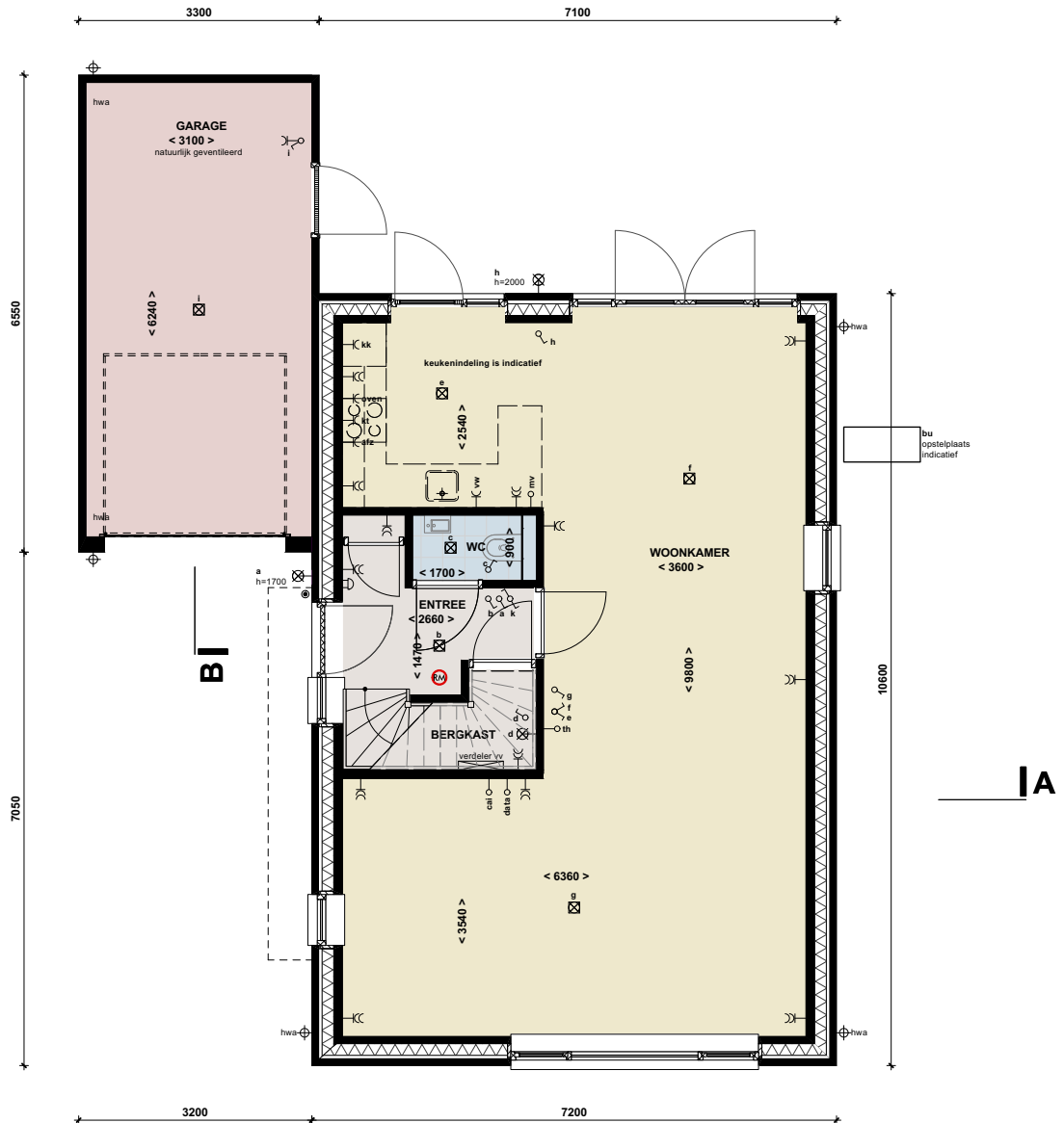
BEGANE GROND type A.2sp schaal 1:100
