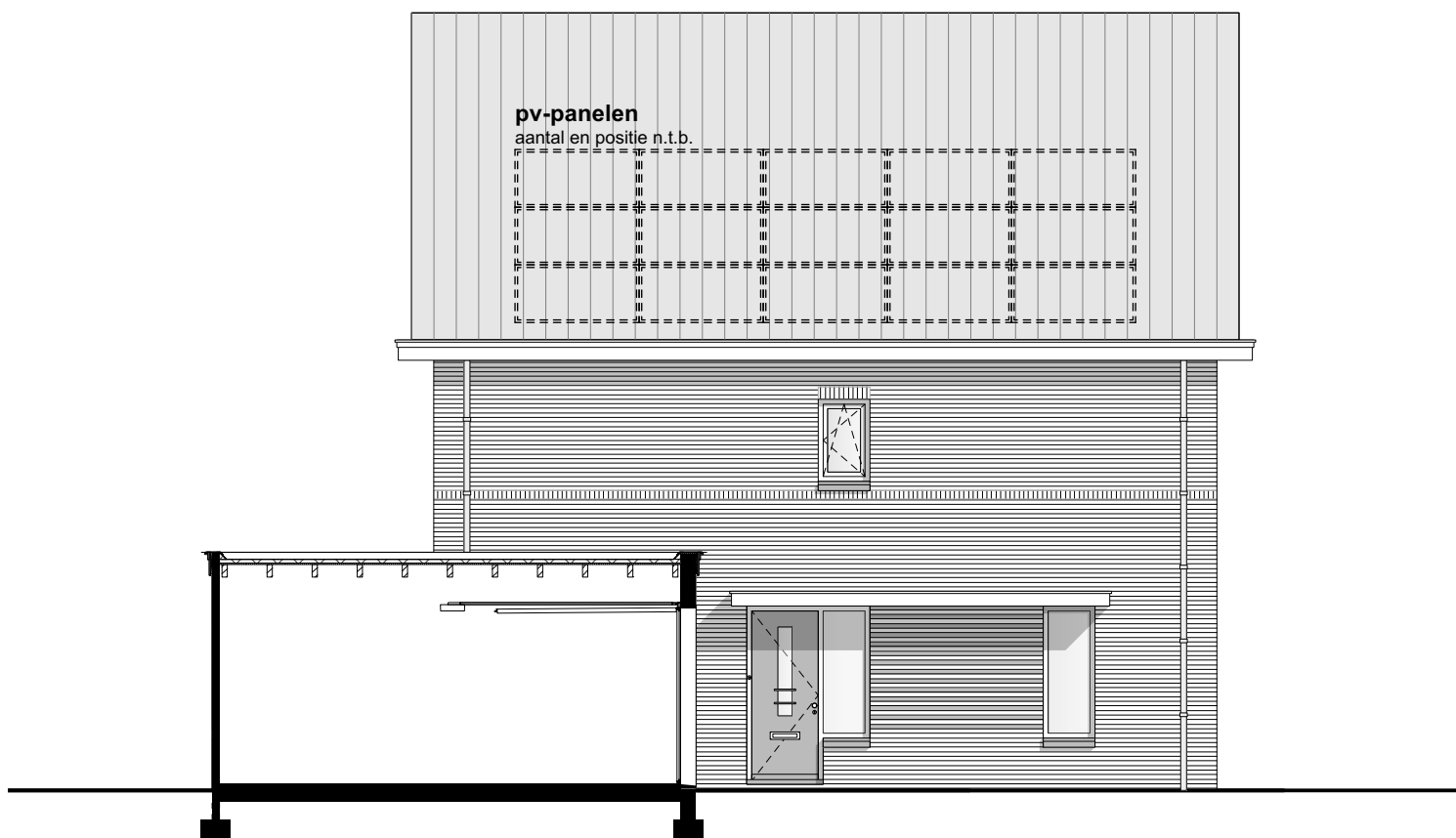
DOORSNEDE B type A.2sp schaal 1:100
