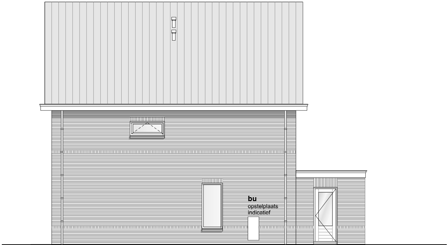
LINKERZIJGEVEL type A.2sp schaal 1:100
