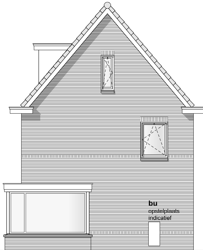
RECHTERZIJGEVEL type B.1 schaal 1:100
