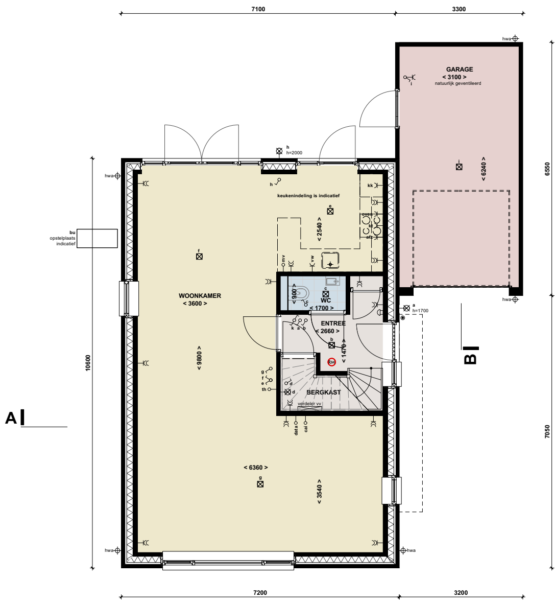
BEGANE GROND type A.2 schaal 1:100
