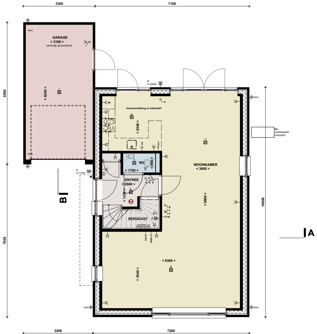
BEGANE GROND type A.1sp schaal 1:100
